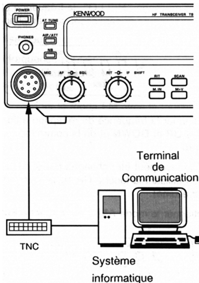
Connecteur MIC et câble de signal TNC
