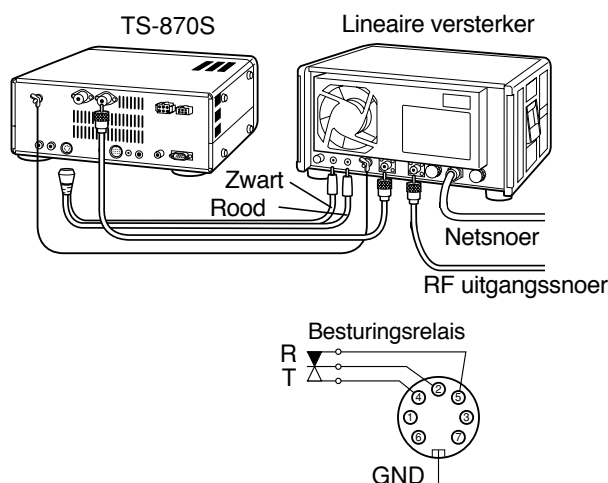
REMOTE aansluiting (Aanzicht vanaf achterpaneel)
